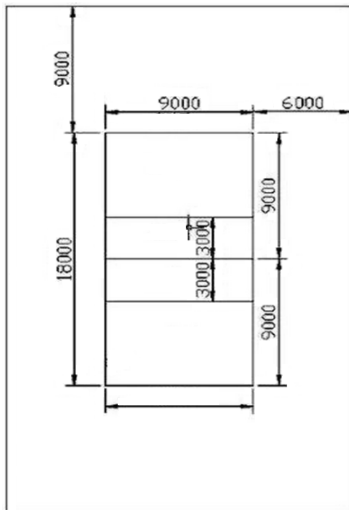
排球比賽場地規格
